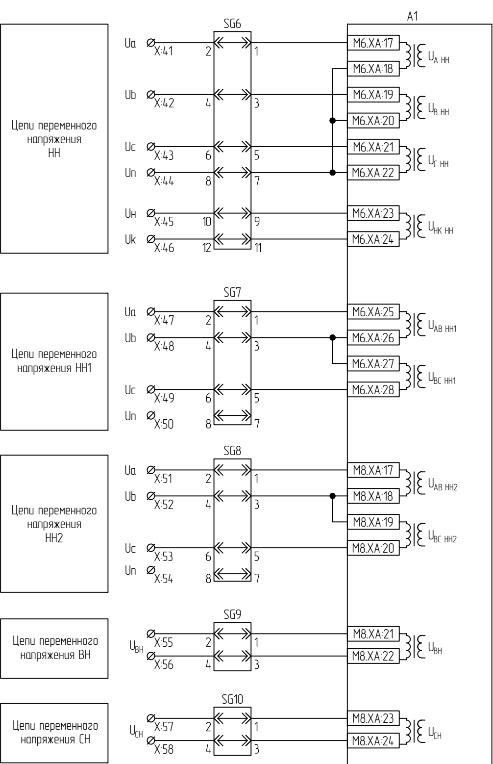
Цепи переменного напряжения
