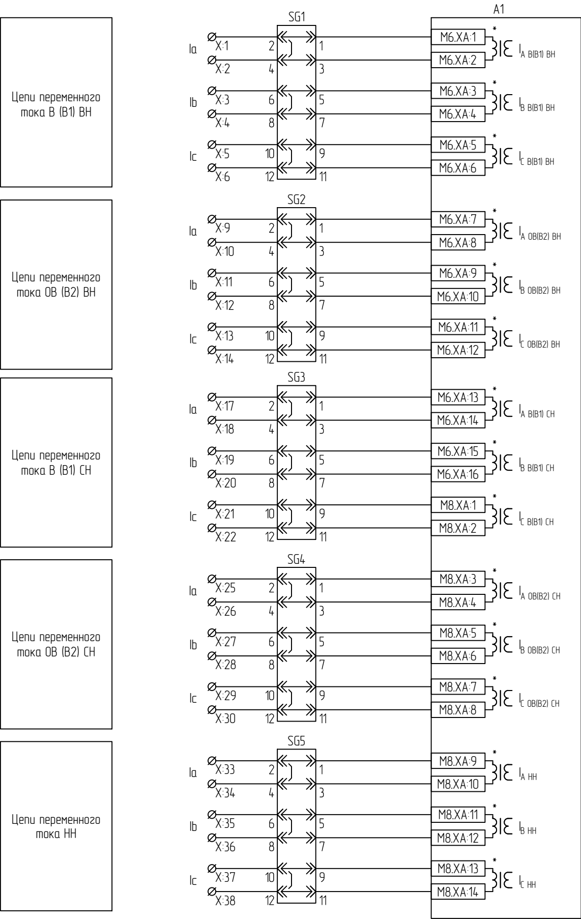
Цепи переменного тока
